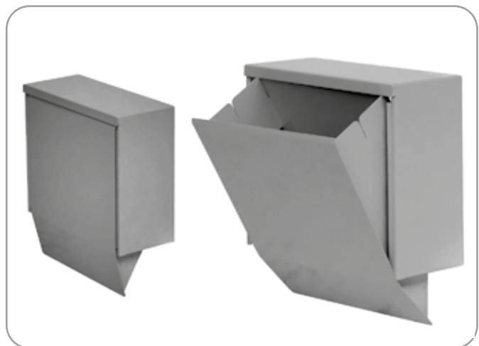
SLIDE15E Abfallbehälter 15 l aus Edelstahl mit Kniebetätigung, Gesamtmaße: 460 x 400 x 170 / 420 x 570 x 210 mm (BxTxH)
